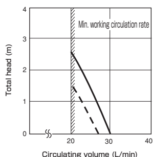
RKS750F / 750F-W
