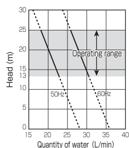
PEC400B1-VW
